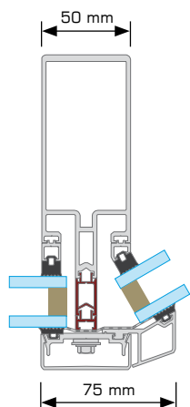
przekrój przez słup kątowny
