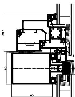
przekrój przez rygiel i okno odchyłne
