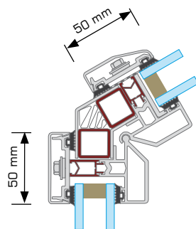
przekrój przez rygiel obrotowy
