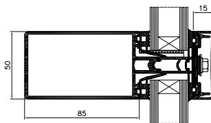
przekrój przez rygiel
