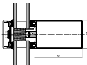
przekrój przez rygiel
